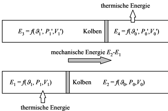
Abb. 2.1. Prinzip einer Dampfmaschine
